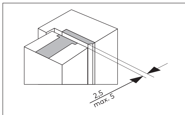
Fig. 20 Vérifier l'entrebâillement
