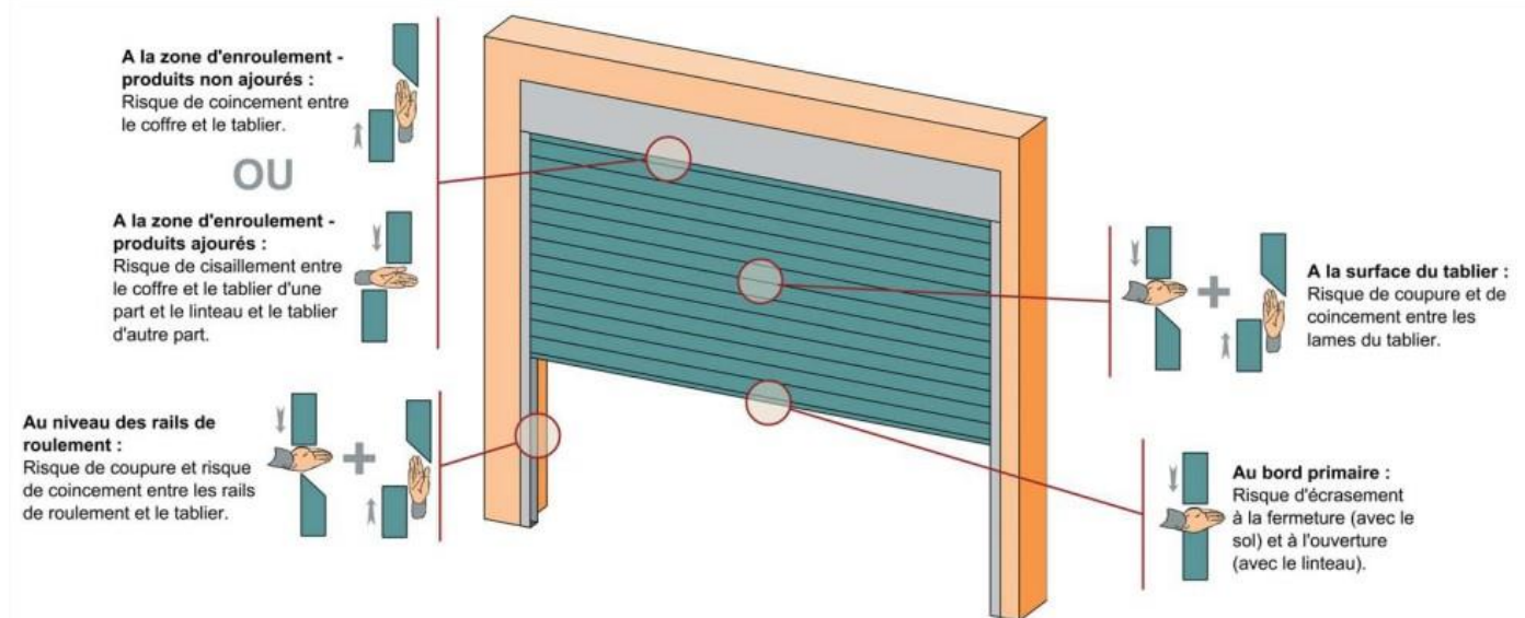
Schéma des principales zones de danger à protéger sur grille et rideau à enroulement
