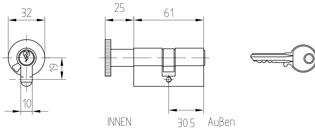
Pos.4 Profil-Zylinder Knopf/Schlüssel
