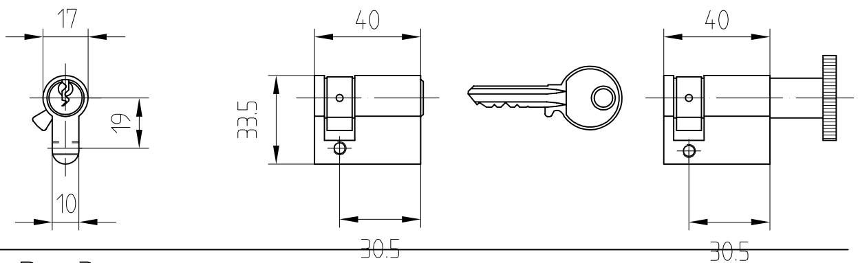
Pos.3 Profil-Zylinder Knopf/Stiftschlüssel
