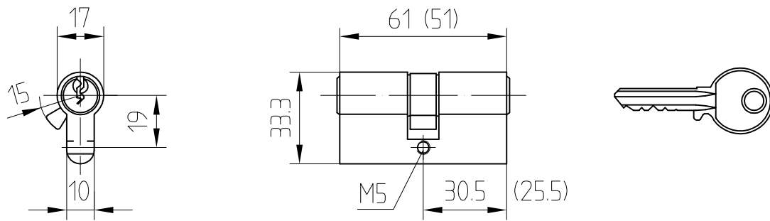
Pos.2 Profil-Zylinder Mitnehmer links/Tür DIN rechts Mitnehmer rechts/Tür DIN links
