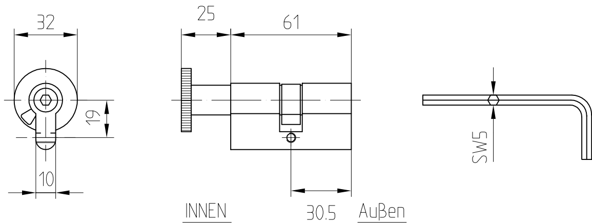
Pos.4 Profil-Zylinder Knopf/Schlüssel
