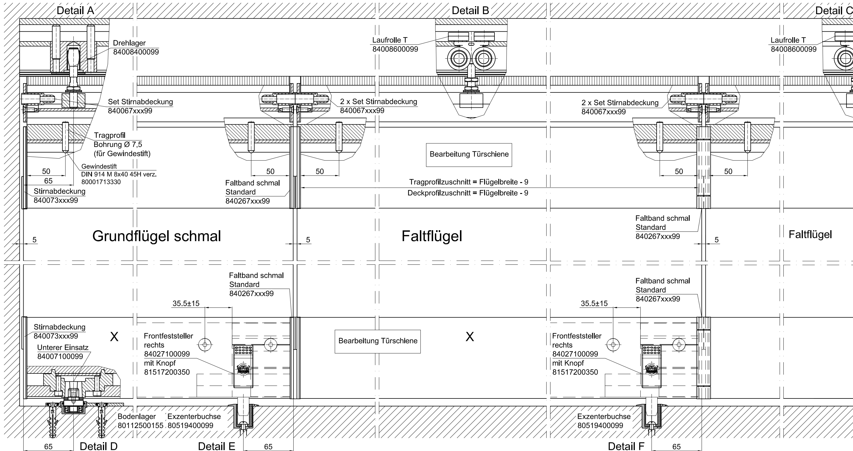
Detail X Bearbeitung Deckprofil, mit 1 Frontfeststeller
