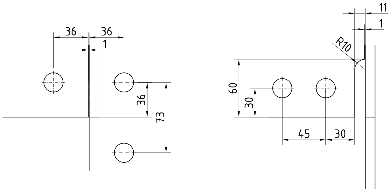
Winkelverbinder mit einseitiger Aussteifung (innen)
