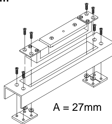
Montage pour portes alu ou PVC
