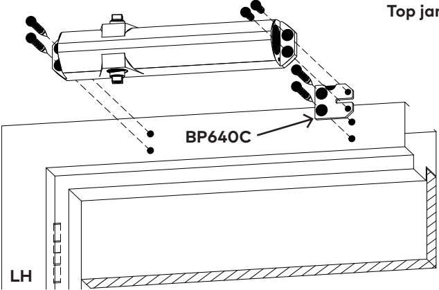
Top jamb mount
