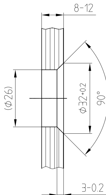
Detail Senkbohrung
