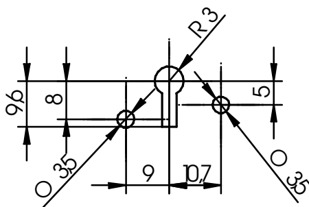
Skizze 1: Befestigungslochbild
