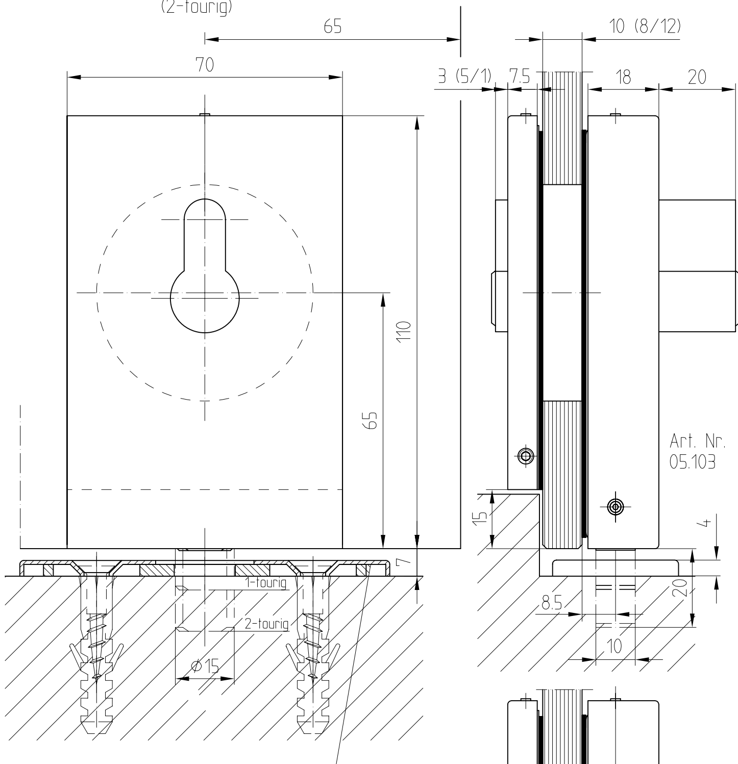
Schließblech Art. Nr. 05.190
