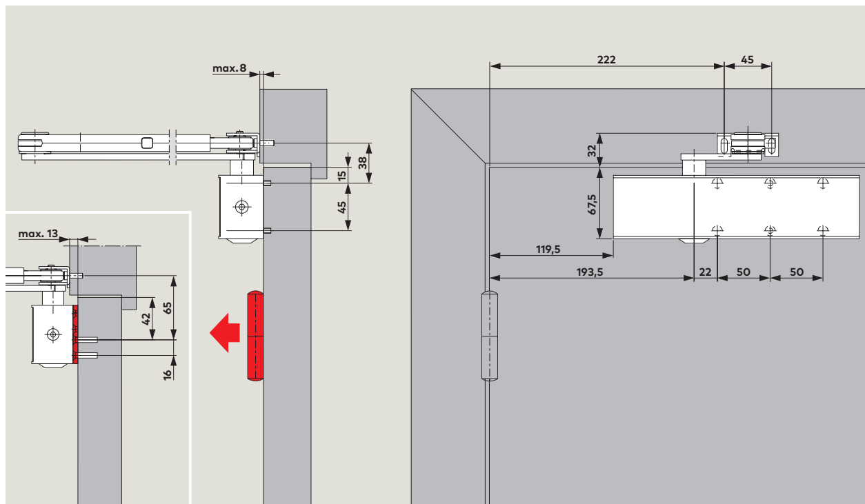
Esempio: porta DIN-SX, porta DIN-DX speculare
