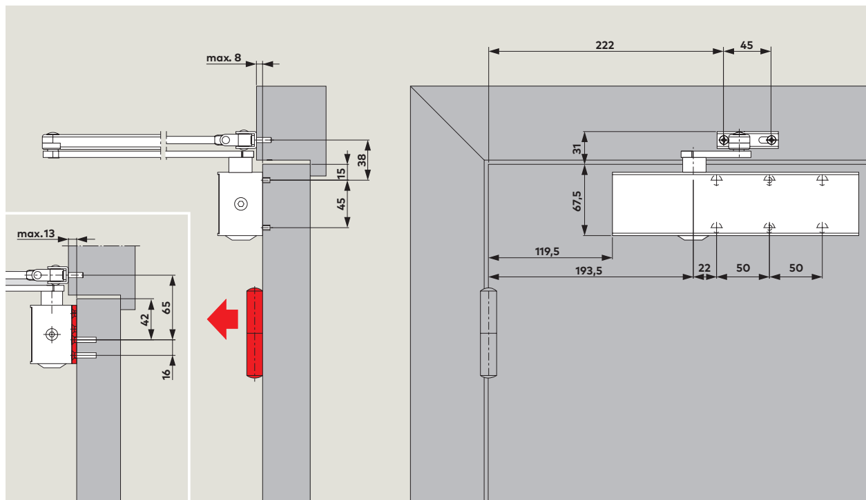
Esempio: porta DIN-SX, porta DIN-DX speculare
