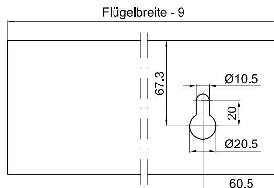
Detail X Bearbeitung Deckprofil, mit 1 Frontfeststeller
