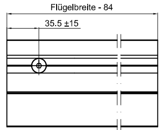
Detail X Bearbeitung Türschiene für Multilock (Maß für erste Bohrung)
