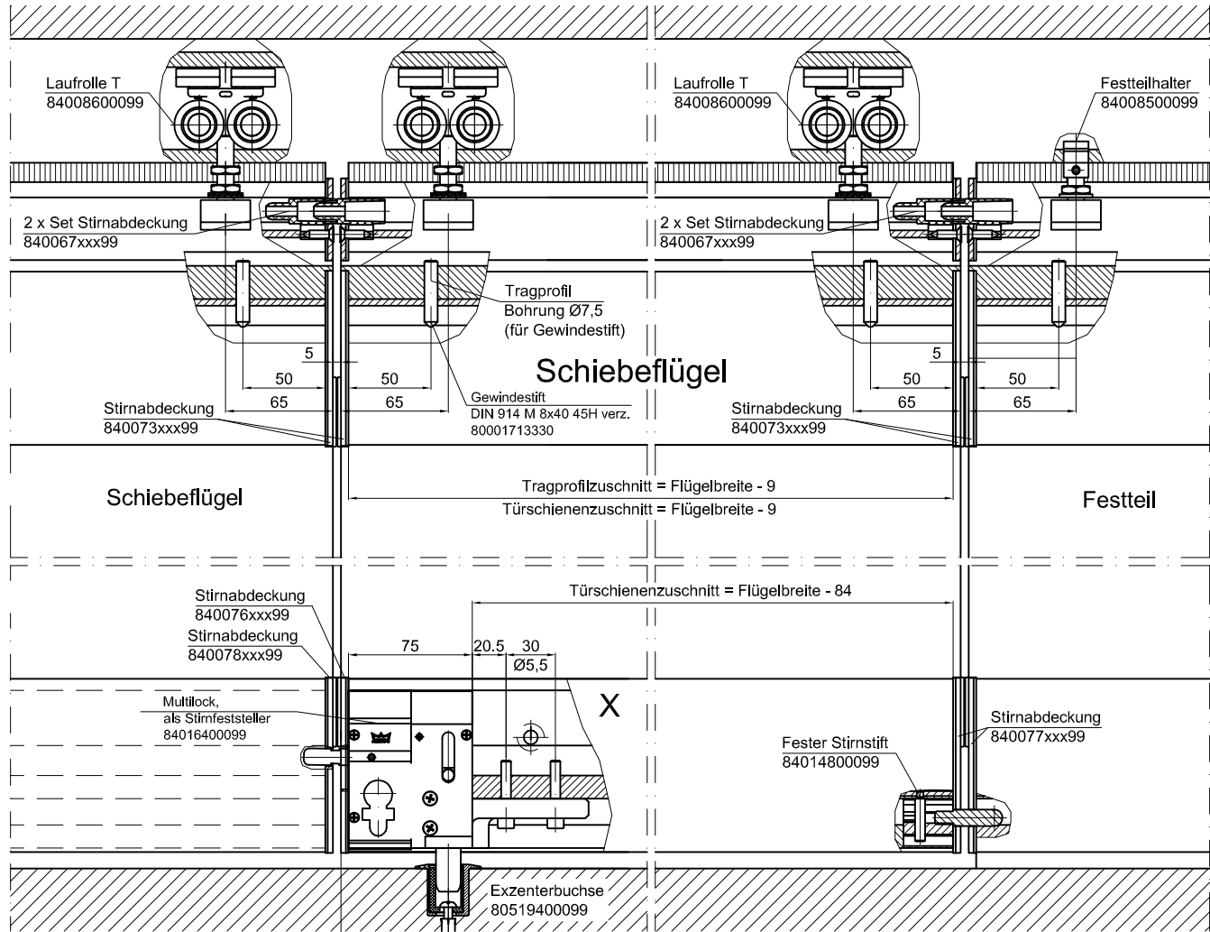
Detail X Bearbeitung Türschiene für Multilock (Maß für erste Bohrung)
