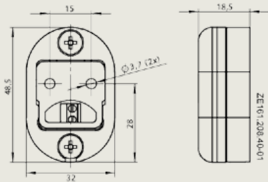
Dimensiones de Kaba Wireless Gateway 90 03 (en mm).
