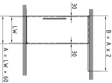
Einzelflügel an Decke
