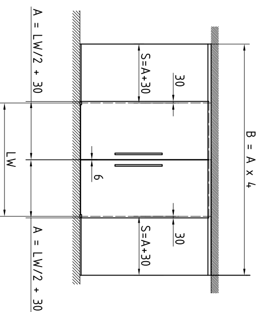
Doppelflügel an Decke mit Seitenteilen
