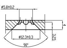
Detail Befestigungsbohrung Laufschiene
