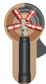
Przekrój poprzeczny klucz Kaba expert/expert Plus
