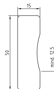
Ausschnitt Stahlzarge
