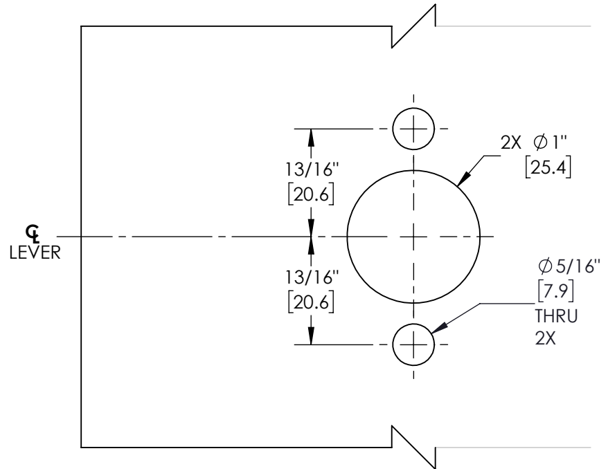
DOOR DETAIL
