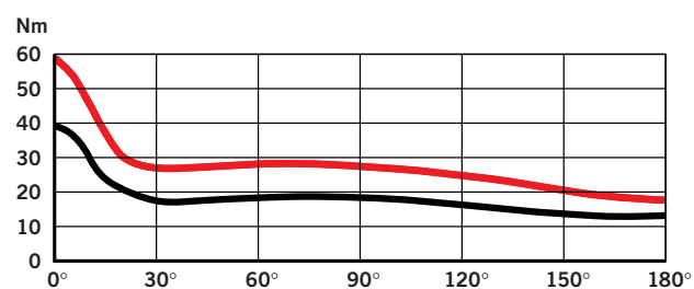
Momentkurve DORMA TS 93 (Lukkekræftinnstilling EN 5)
