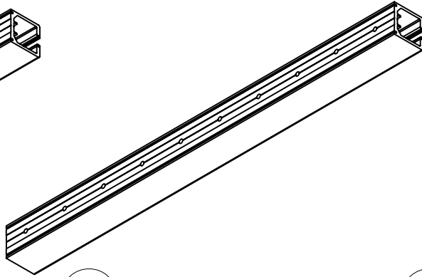
2 Laufschiene mit 100er Bohrungsabstand Z.-Nr. 8.15.241.002.40 Art.-Nr. 15.593
