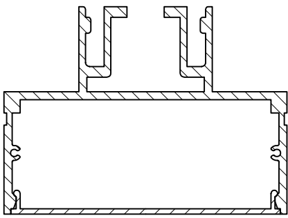
↑ Ansicht X
