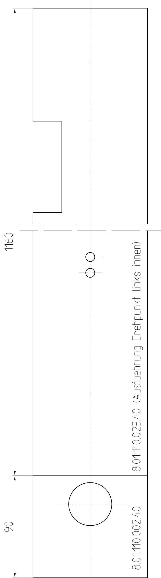
Ansicht X
