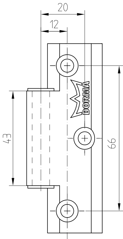
Ansicht Rahmenteil
