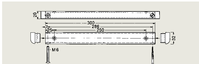
Glissière Réf. art. 7453 N
