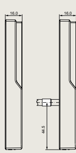
dormakaba Kompaktleser 91 04, Seitenansicht; IP66-Ausführung mit Kabelabgang
