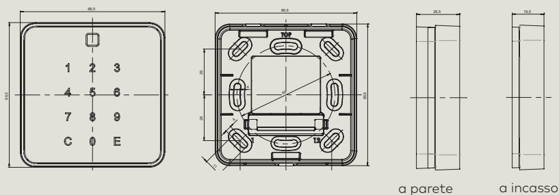
Unità di rilevamento dormakaba 90 02 Pannello frontale e posteriore
