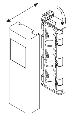
4002 Portabaterías grande con alarma
