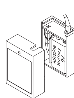
2788 Portabaterías pequeño o 2789 Portabaterías pequeño con alarma
