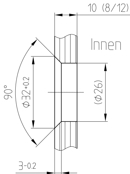
Detail Senkbohrung (1:1)
