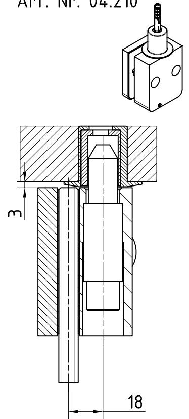
Deckenverriegelung TA-Tür mit Schließung in Buchse Art. Nr. 04.210
