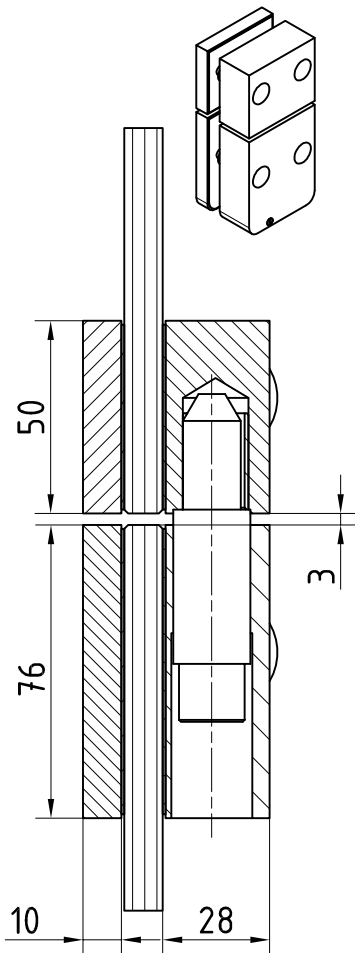
Pendeltür Art. Nr. 04.207
