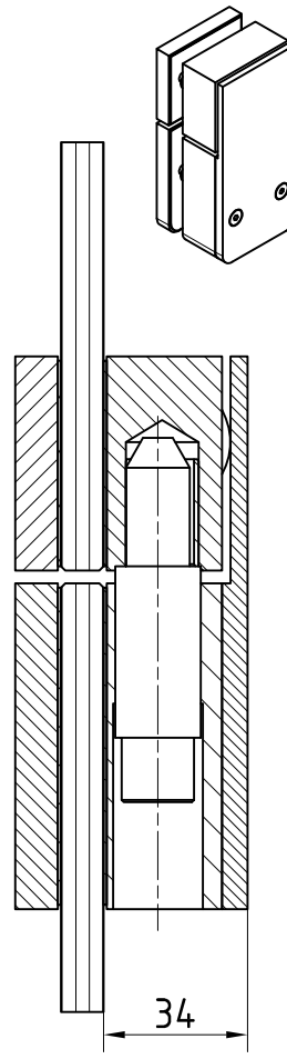
TA nach innen öffnend Art. Nr. 04.209
