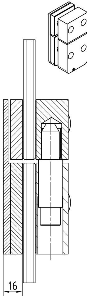
TA nach ausssen öffnend Art. Nr. 04.208
