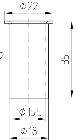
Bodenbuchse mit Stopfen Art. Nr. 05.193
