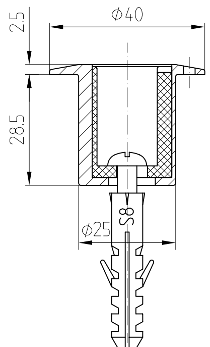
Exzenterbuchse Art. Nr. 05.194
