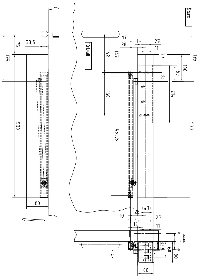
Sturzmontage Bandseite DIN links Sturzmontage Bandseite DIN rechts: spiegelbildlich
