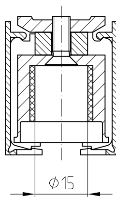
Coupe A-B
